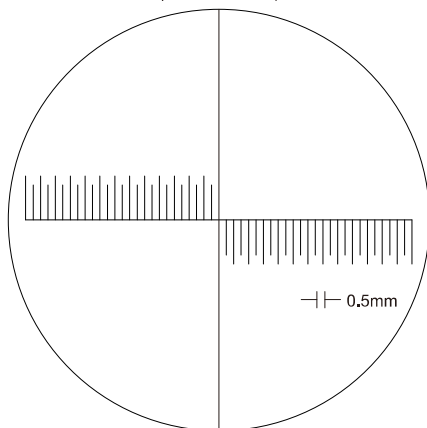
7527-D1底板刻线 (分度值0.5mm)
