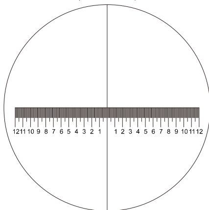
7527-D1B底板刻线 (分度值0.1mm)
